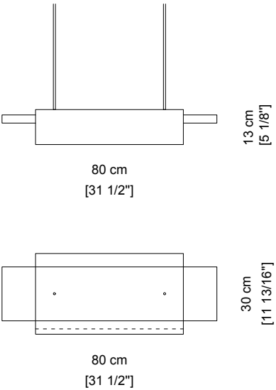
Dimensions
